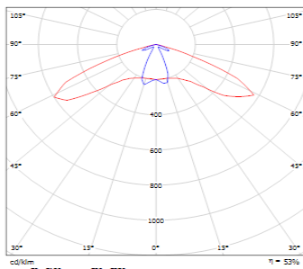
Curva fotométrica
