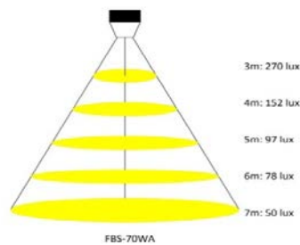
Iluminación Estimada
